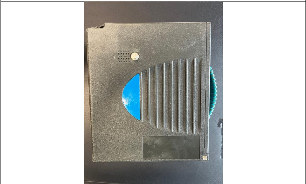
32. Seitenansicht beider Geldkassetten Hersteller: JCM, Model: UBA
